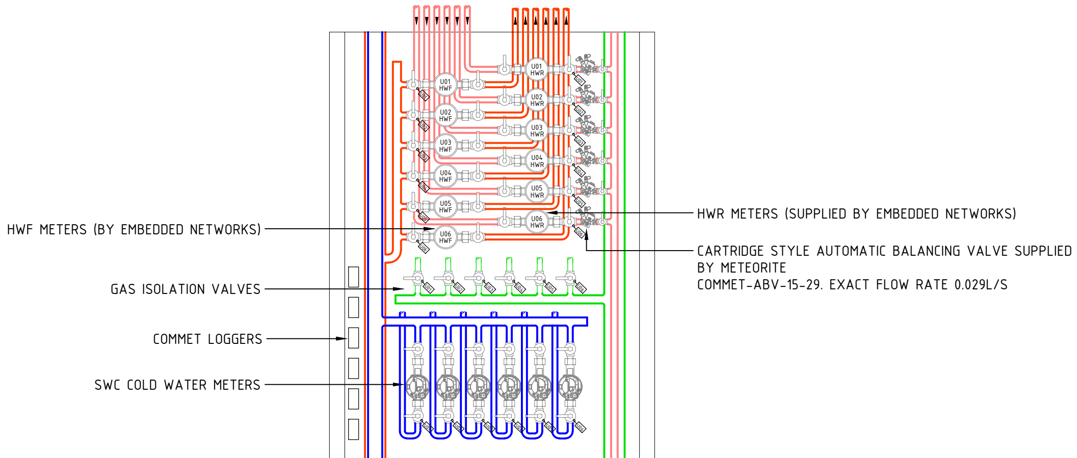
ELEVATION
